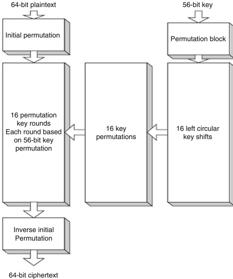
Fig. 11.3 DES algorithm
